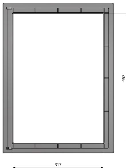
DIMENSIONI DI ACCESSO ALLA NICCHIA
