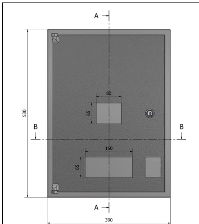
INGOMBRO ESTERNO
